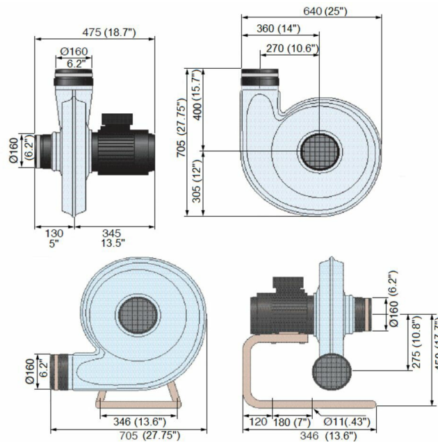
Wentylator N 29, wersja ze stojakiem i bez
